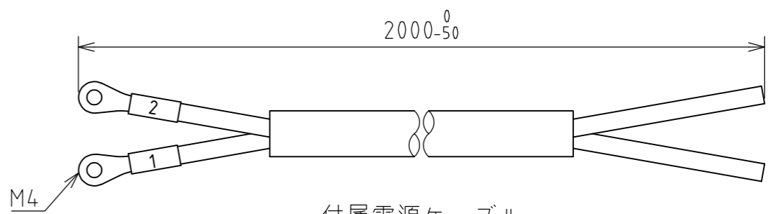
付属電源ケーブル (2.0sq キャブタイヤ 2芯)
