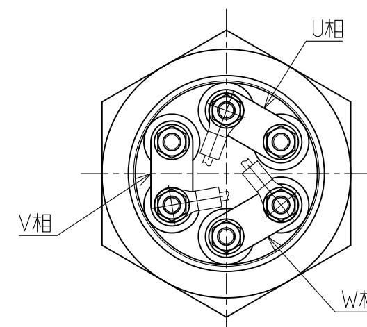
ヒータ結線例
