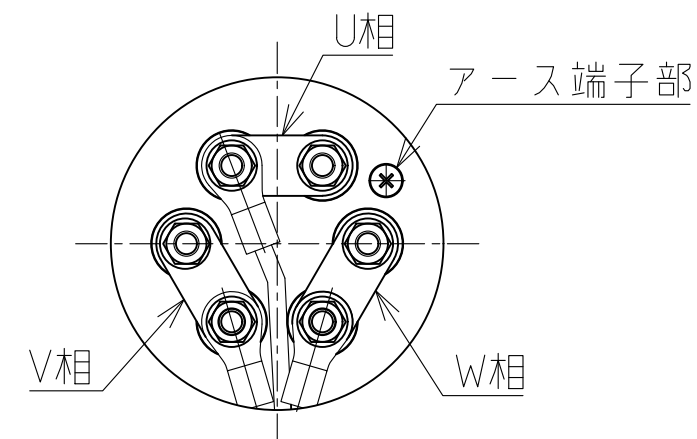
ヒータ結線例
