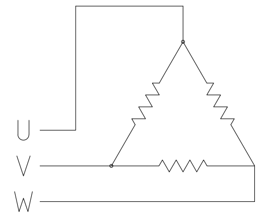
回路図
