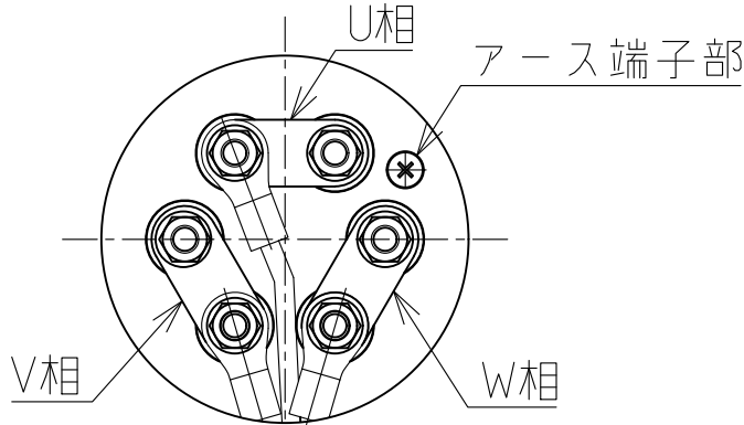
ヒータ結線例
