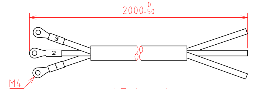
付属電源ケーブル (5.5sq キャブタイヤ 3芯)
